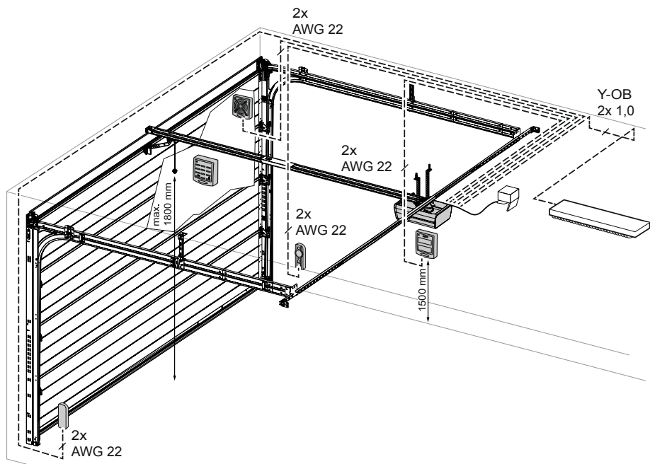
Abb. 3: Beispielinstallation Zubehör
