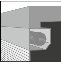
Pose en tunnel, enroulement intérieur
