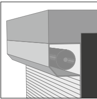
Pose en tunnel, enroulement extérieur
