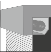
Pose en applique intérieure
