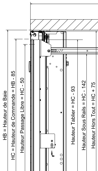
Disposition B : pose en tunnel
