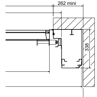
Coupe horizontale : effacement derrière écoinçons
