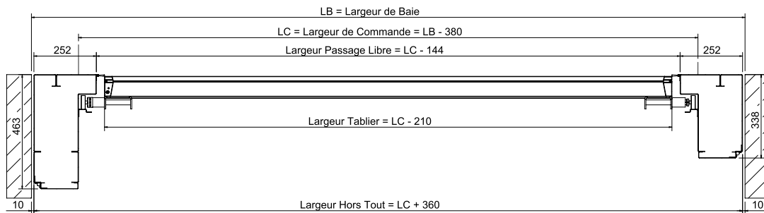
Coupe horizontale pose en tunnel
