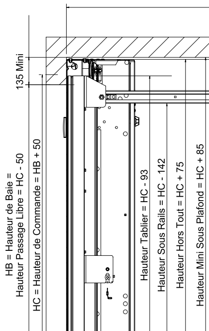
Disposition C : effacement derrière linteau
