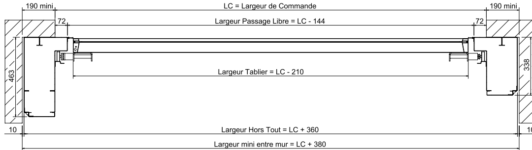
Coupe horizontale pose en applique
