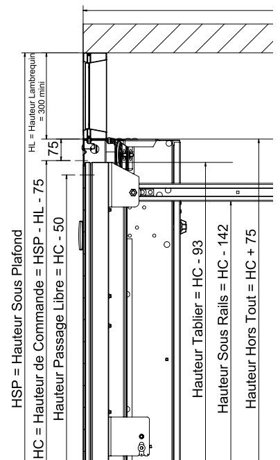
Disposition D : pose sous lambrequin
