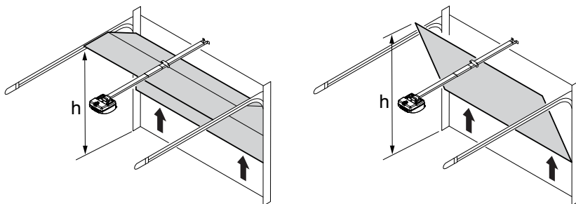
Fig. 5: Mesure de la hauteur totale de la porte de garage
