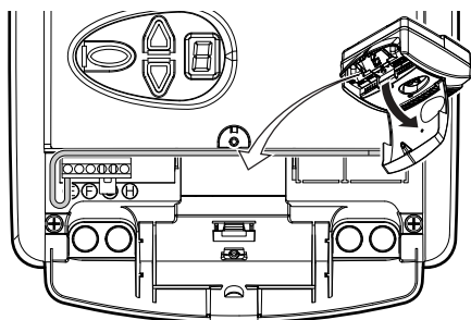
Fig. 7: Ouverture du couvercle de la tête de commande et d'entraînement
