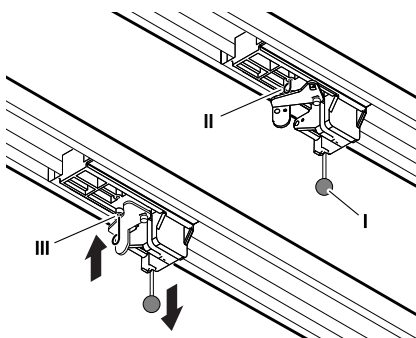
Fig. 6: Déverrouillage et verrouillage de l'entraînement
