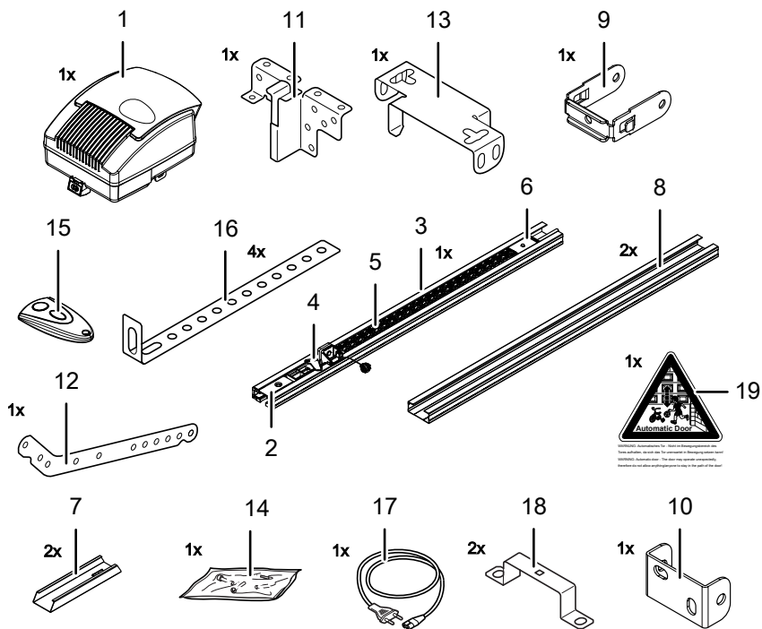
Fig. 4: Composition de la fourniture
