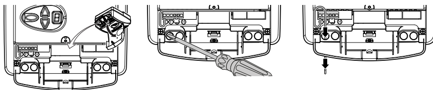
Fig. 8: Poser l'antenne
