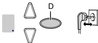
Fig. 11: Effacement de tous les émetteurs portatifs programmés sur la tête d'entraînement
