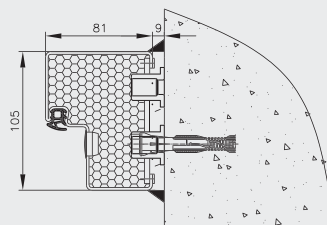
BÂTI TUBULAIRE
