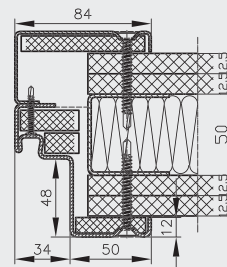
BÂTI 2140B
